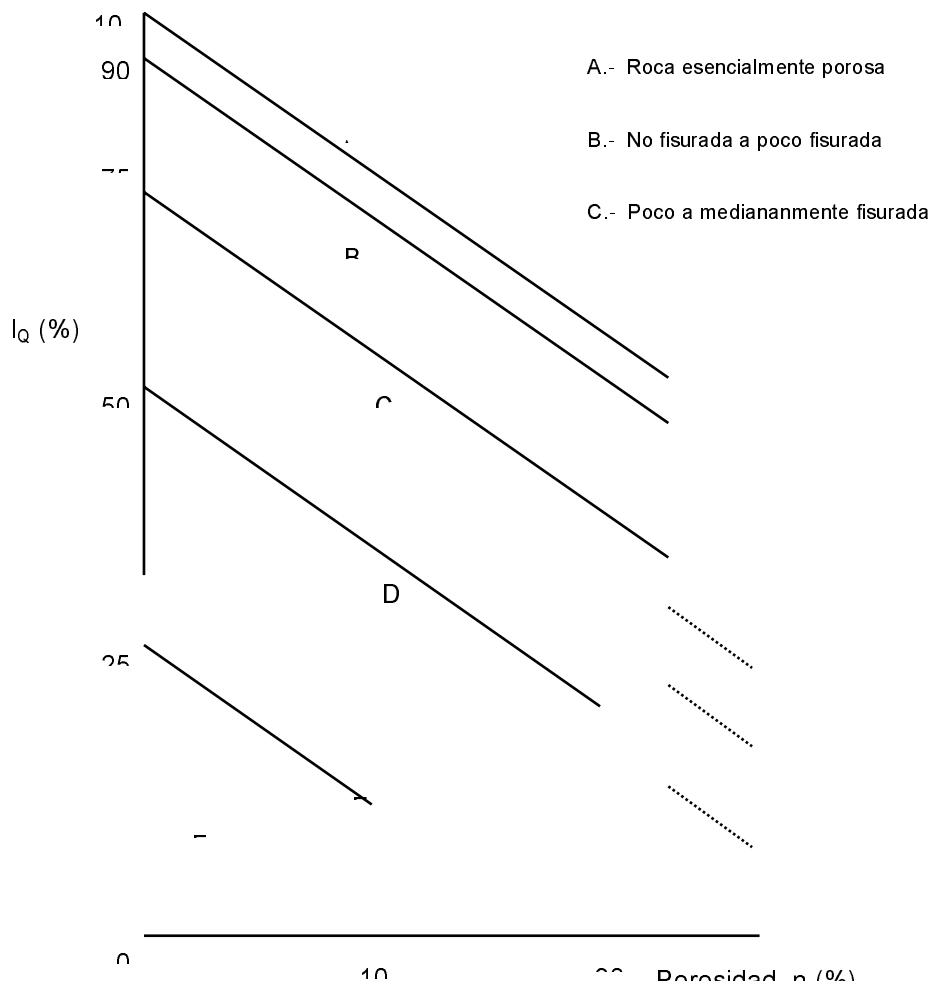
Fig. 6.2. Descripción de la densidad de fisuración de una muestra de roca con ayuda del índice de calidad y la porosidad total. (modificado de FOURMAINTREAU, 1976; en OTEO MAZO, 1978).
