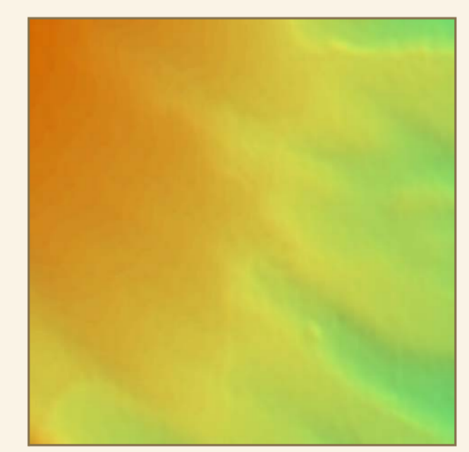
HIPSOMETRÍA DE LA HOJA
