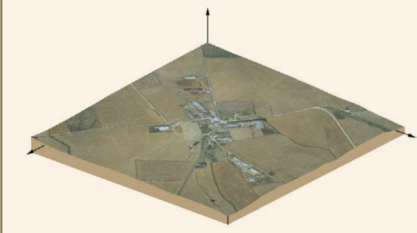
HIPSOMETRÍA DE LA HOJA
